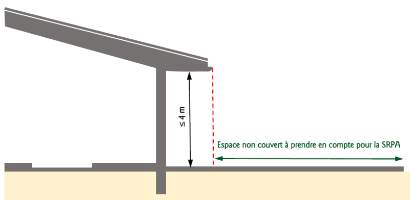
Fig. 1 : Principe de mesure pour des avant-toits de 4 mètres et moins
