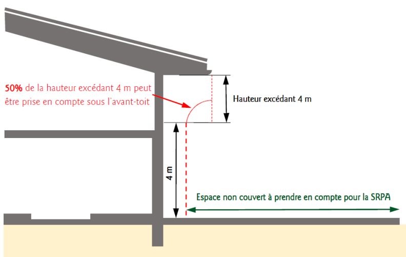
Fig. 2 : Principe de mesure pour des avant-toits de plus de 4 mètres
